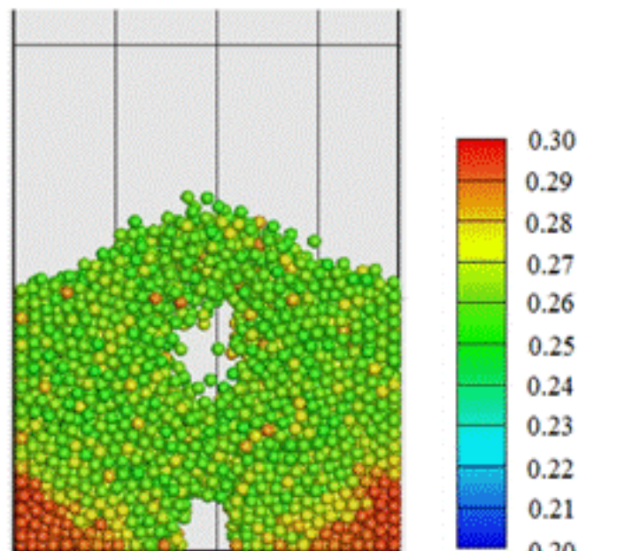
含水粒子の乾燥モデル
