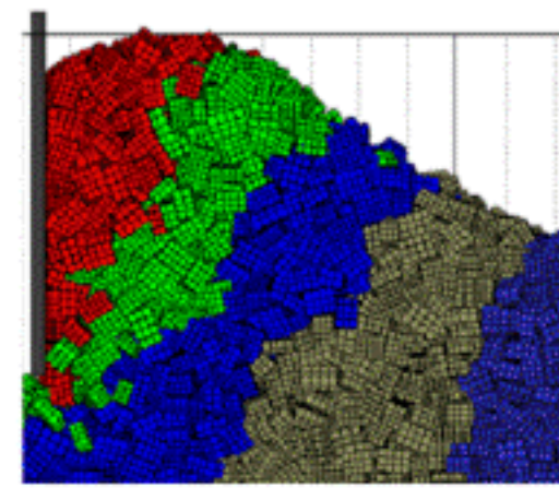
非球形粒子モデル
