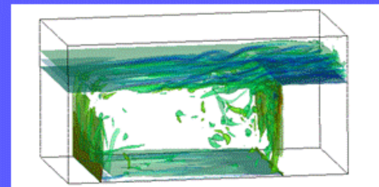
底面速度-0.34の渦度
