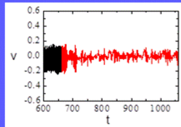
底面速度-0.34の振動
