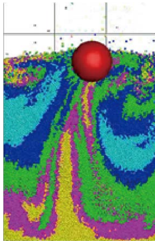
サイズが大きく異なる 固体群の運動モデル
