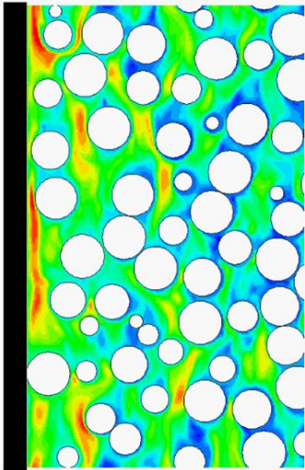
高濃度に固体粒子を含む 流れ場の直接数値計算
