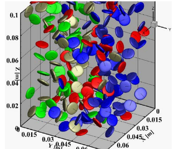
非球形粒子モデル
