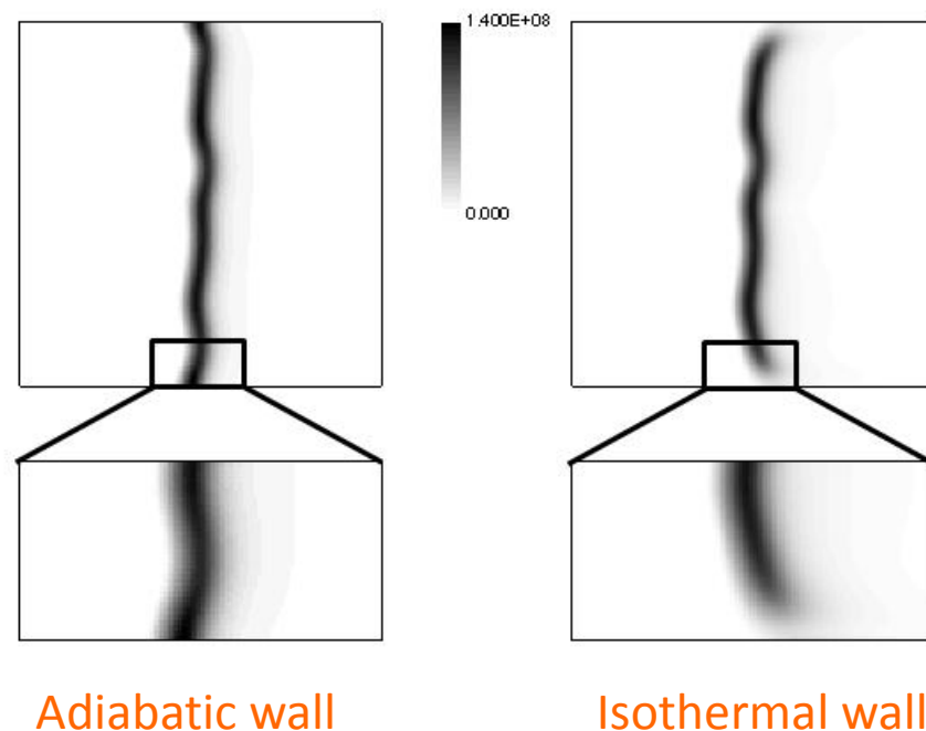
Fig. 1 壁面近傍の化学的過程を考慮した水素-空気乱流予混合火炎の熱発生率分布。断熱壁(左)と等温壁(右)
