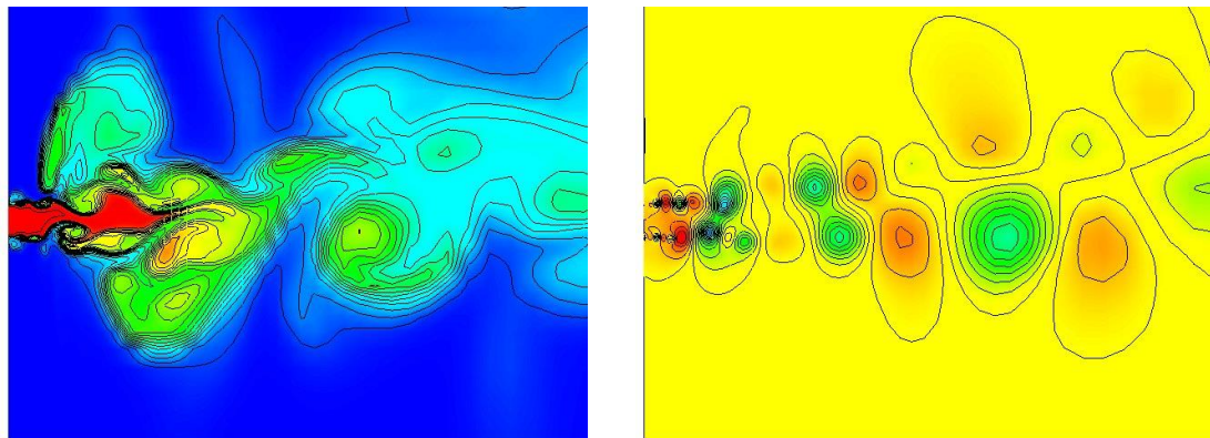
図1. 低速水素噴流の計算結果. 左: 瞬間密度分布, 右: 瞬間圧力分布
