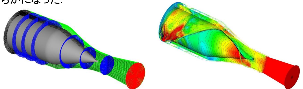
図1. 回転デトネーションエンジンの計算結果. 左: 計算格子, 右: 瞬間マッハ数分布
