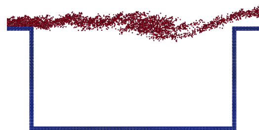
図 せん断層で生成した渦構造
