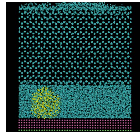
壁面近傍の凝固過程
