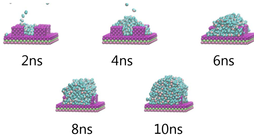
ナノ構造が凝縮過程に及ぼす影響
