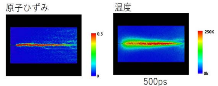
図：分子動力学シミュレーションにおける亀裂成長と温度上昇の様子(500ps時)。
