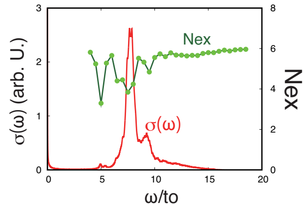
図. \sigma(\omega) : 光学電気伝導度、 N_{ex} : 粒子励起数。 \omega は振動数で、 t_0 は単位とするエネルギースケール。
