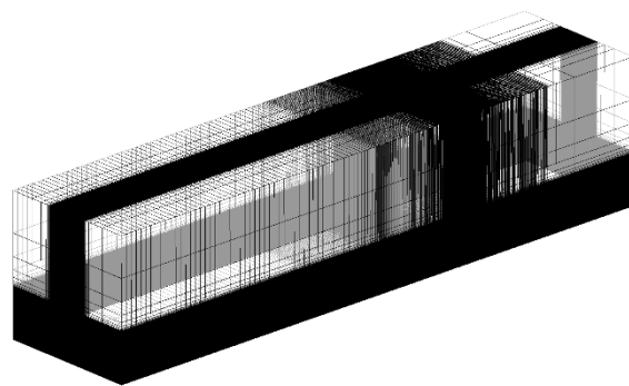
図1. 超音速流と垂直水素噴流の干渉の計算結果。 左：計算格子，右：断面瞬間温度分布
