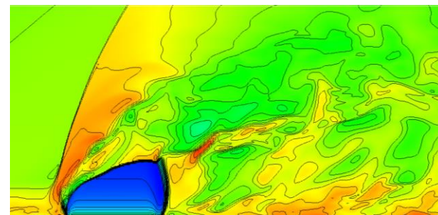
図1. 超音速流と垂直水素噴流の干渉の計算結果。 左：計算格子，右：断面瞬間温度分布
