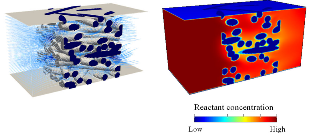
多孔質電極における電気化学反応輸送解析結果
