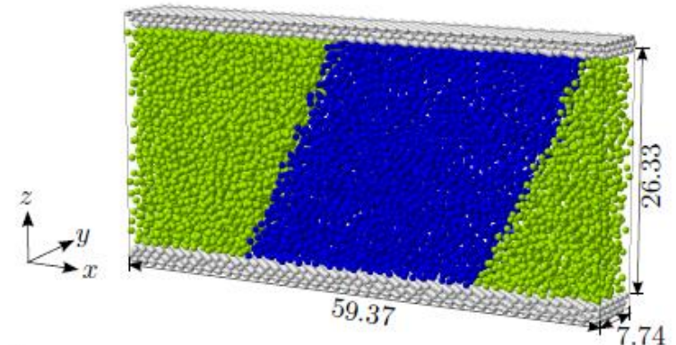
不溶性2液流の分子動力学計算例
