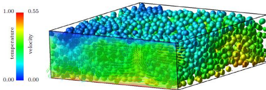
固液二相対流伝熱の差分計算例
