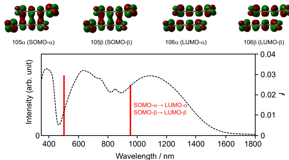
図 1. TCNQ 塩ラジカルアニオンダイマーの TDDFT 計算の結果
