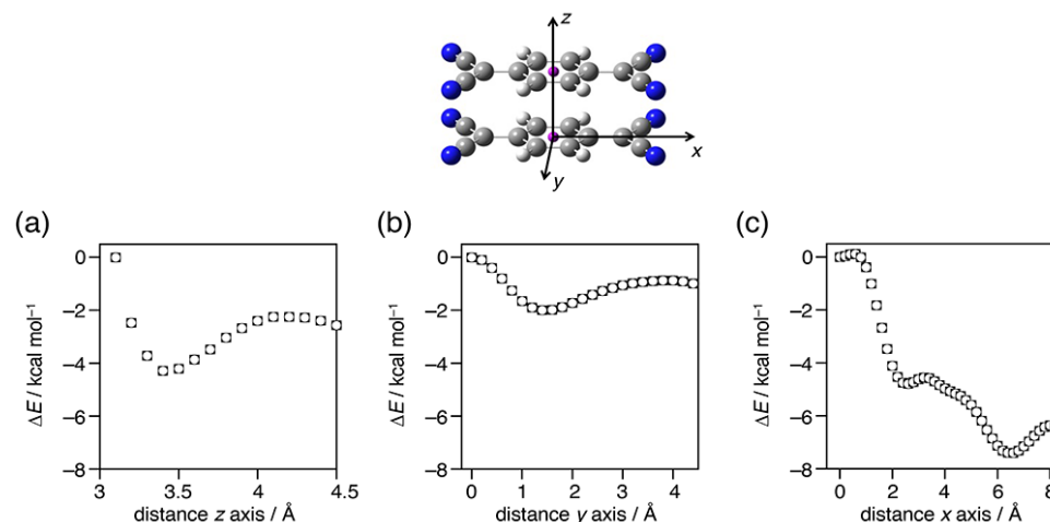
図 1. TCNQ ラジカルアニオンダイマーの DFT 計算の結果
